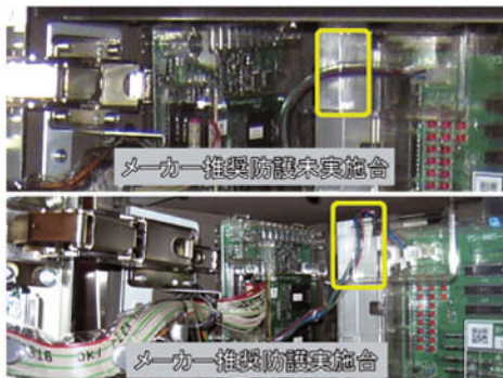
写真3 「豪炎高校」 メーカー推奨防護実施例
