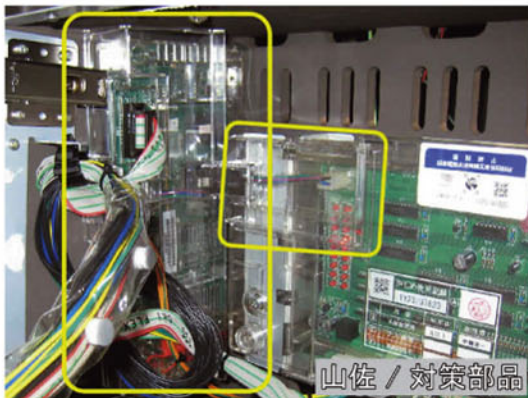
電源経路
