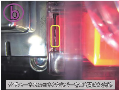
サブハーネスのコネクタカバーをこじ開けた痕跡
